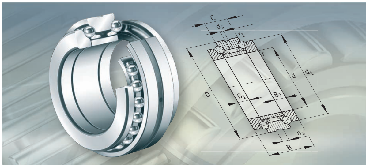
Rodamientos axiales de bolas de contacto angular
