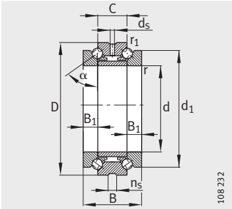
2344, 2347 Ángulo de contacto \alpha = 60^\circ
