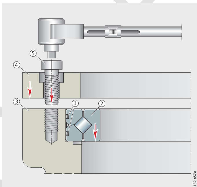
Figura 9 Fijación del anillo exterior
