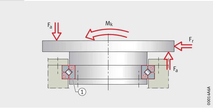
Figura 2 Rodadura con un rodamiento de rodillos cruzados
