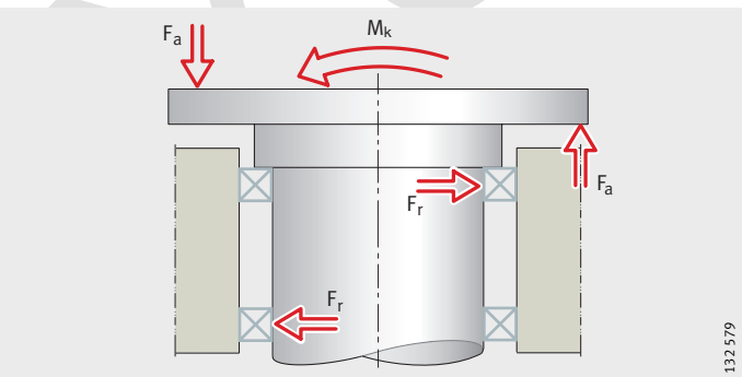
Figura 1 Rodadura clásica con dos rodamientos
