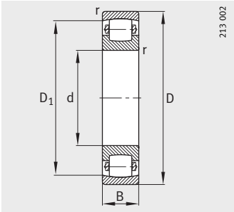
Agujero cilíndrico
