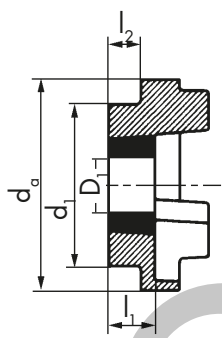
F flange
