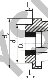
H flange
