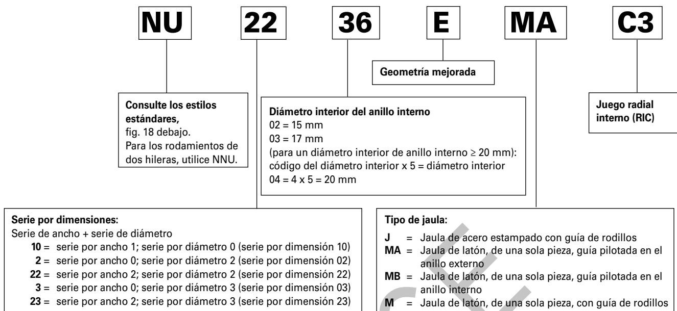
Fig. 17. Nomenclatura de rodamiento de rodillos cilíndricos radiales, sistema métrico ISO.
