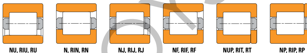
Fig. 18. Estilos de rodamiento de rodillos cilíndricos estándar, en pulgadas y en sistema métrico.
