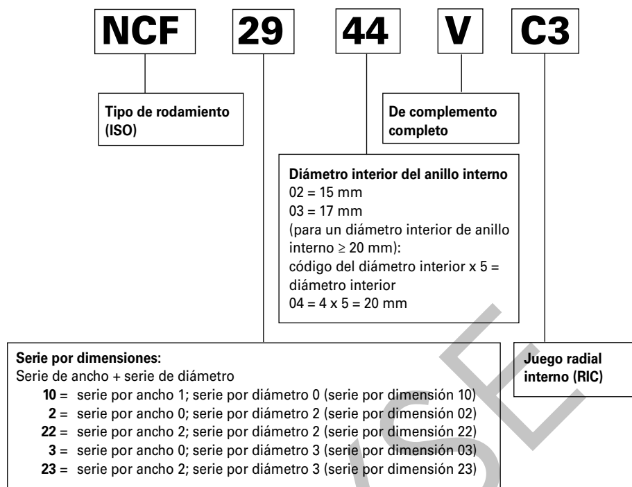
Fig. 20. Nomenclatura para rodamiento de rodillos cilíndricos de complemento completo (NCF).
