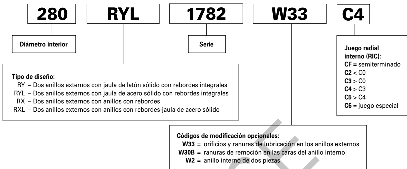
Fig. 38. Nomenclatura del conjunto de rodillos cilíndricos de cuatro hileras.
