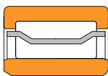
Fig. 3. Jaula tipo S.
