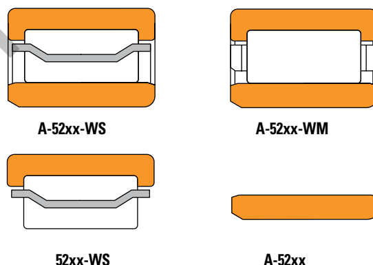
Fig. 2. Rodamientos de la serie de sistema métrico 5200
