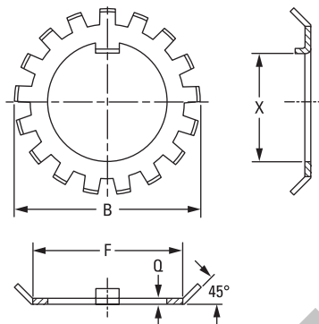
Fig. 50. Arandelas de retención.
