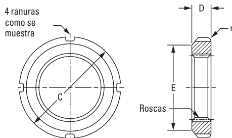
Fig. 52. Tuercas de fijación (las roscas son ISO 965/1, clase 5H).
