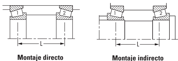
Fig. 16. Montajes directo e indirecto.
