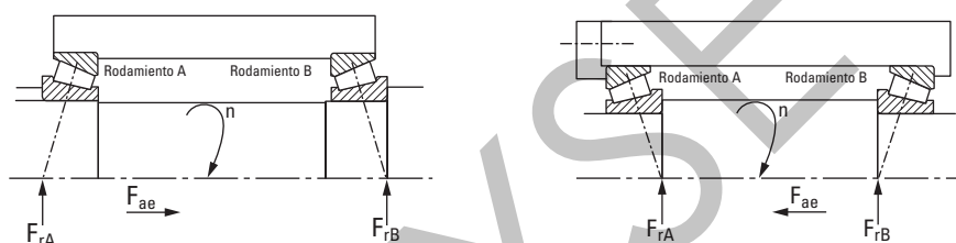
Diseño (carga axial externa, F_{ae} , sobre el rodamiento A)
