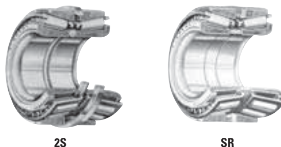
Fig. 6. Conjuntos espaciadores.
