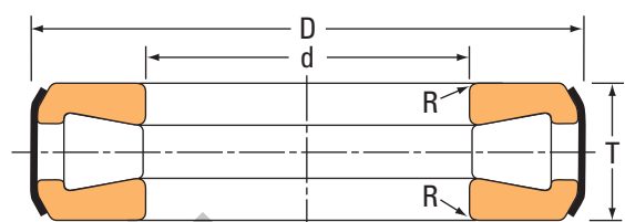
Fig. D. Tipo TTCS.
