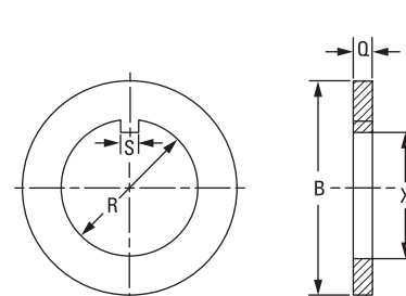
Fig. 54. Arandelas de lengüeta.
