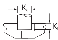
Perno de fijación para rodadura externa de CD.
