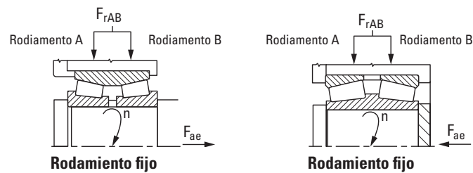
Diseño (carga axial externa, F_{ae} , sobre el rodamiento A)
