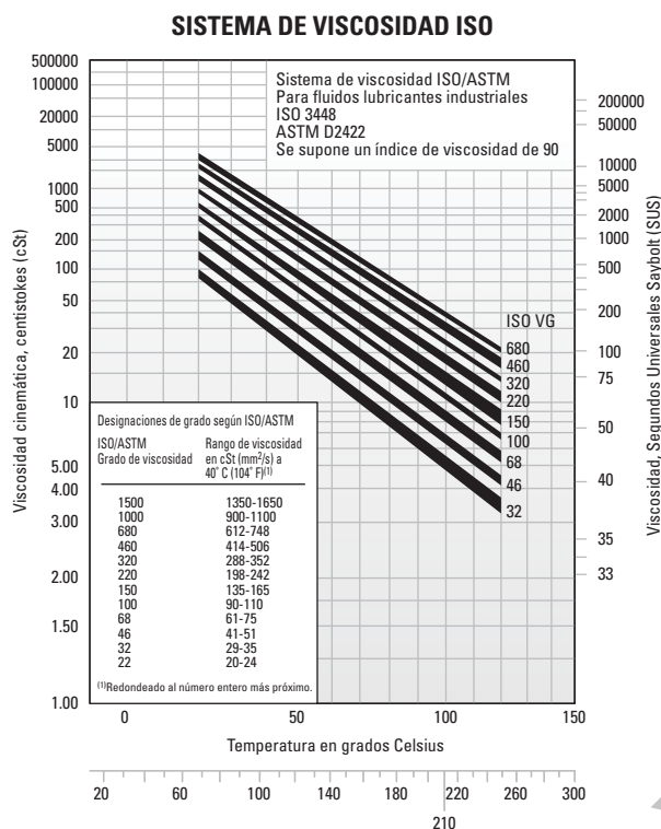
Fig. 22. Sistema de grados de viscosidad para aceites industriales.
