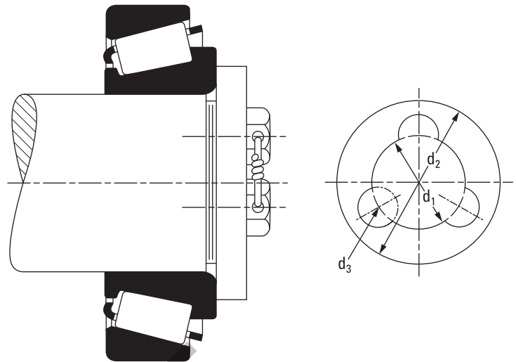
Fig. 58. Cuñas cónicas.
