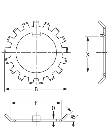
Fig. 53. Arandelas de retención.
