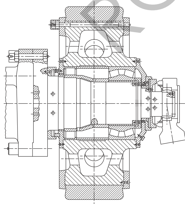
Fig. 12. Ensamble pulverizador de ruedas.
