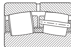
Fig. 10. Jaula con pasador.
