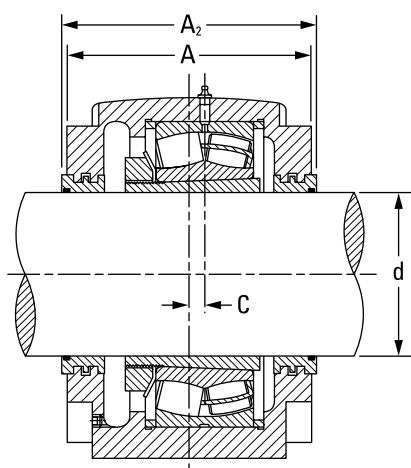
Retén de laberinto
