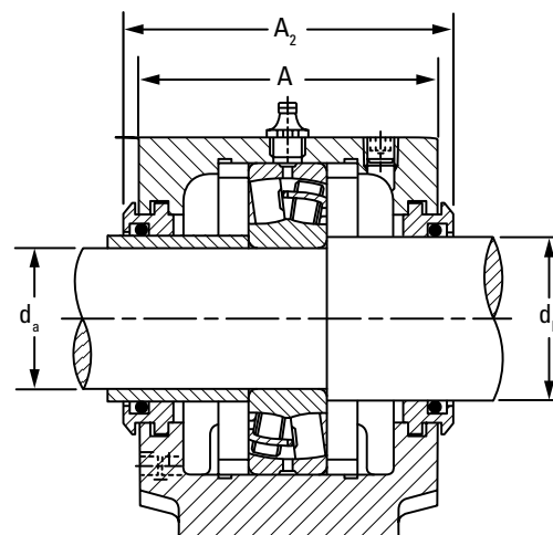
Retén de laberinto
