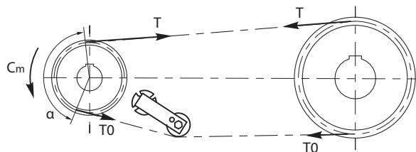
Fig. 6 TENSIONAMENTO DALL'INTERNO VERSO L'ESTERNO TENSIONING FROM INSIDE TO OUTSIDE SPANNUNG VON INNEN NACH AUSSEN TENSION DE L'INTÉRIEUR VERS L'EXTÉRIEUR TENSADO DESDE EL INTERIOR HACIA EL EXTERIOR
