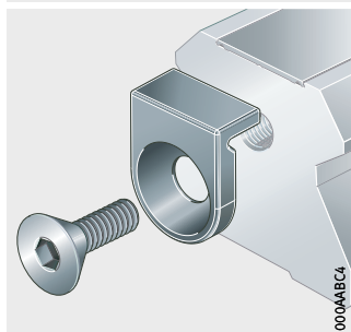
BKE.TSX...-D
