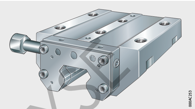
RUKS...D-A-SR
