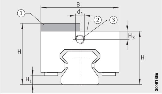
BKE.TSX...-D
