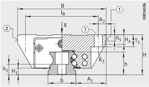
KUE...-B-E
