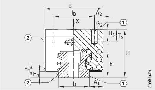
KUSE...-H, KUSE...-HL
