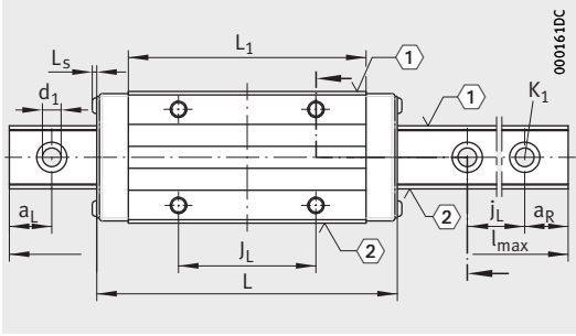
KUVE...-B-HL, KUVE...-B-SL, KUVE...-B-SNL View X rotated 90°
