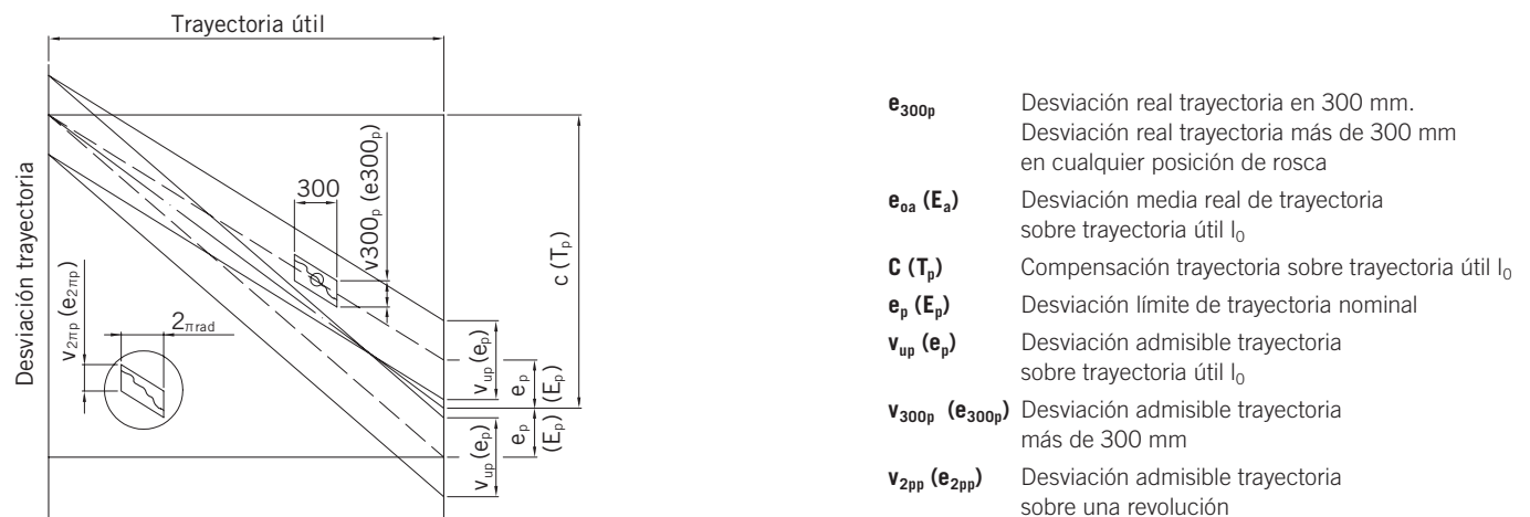
Fig. 3.11 Medición ISO DIN curva de paso del husillo de bolas
