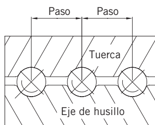
Fig. 3.16 Precarga por tamaño de la bola
