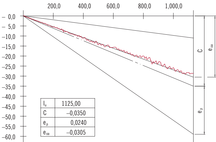
Fig. 3.13 Desviación media trayectoria sobre trayectoria útil l_u
