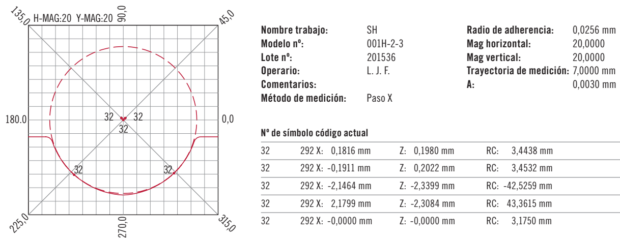
Fig. 2.3 Perfil del arco de la bola probado por HIWIN
