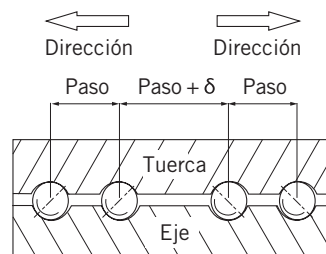
Fig. 3.17 Precarga por compensación del paso
